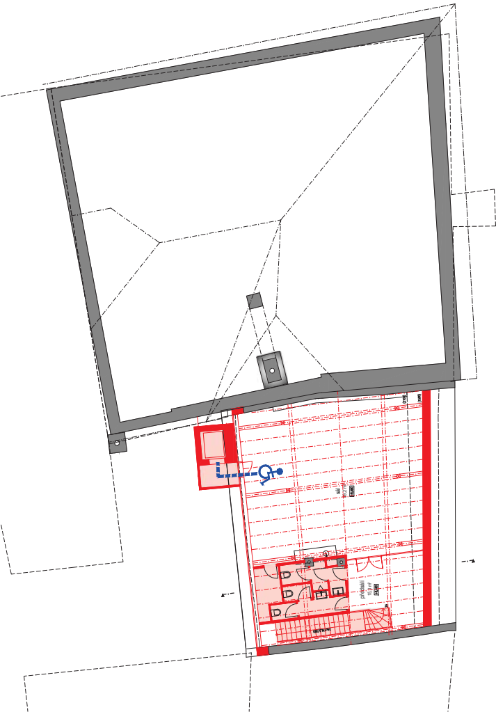
Půdorys - podkroví
